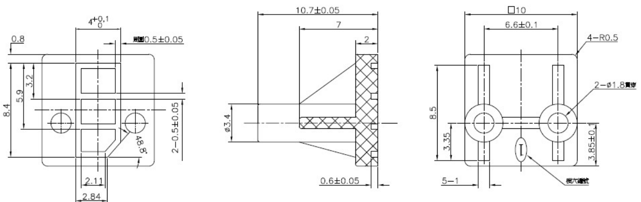
△蓋板尺寸
