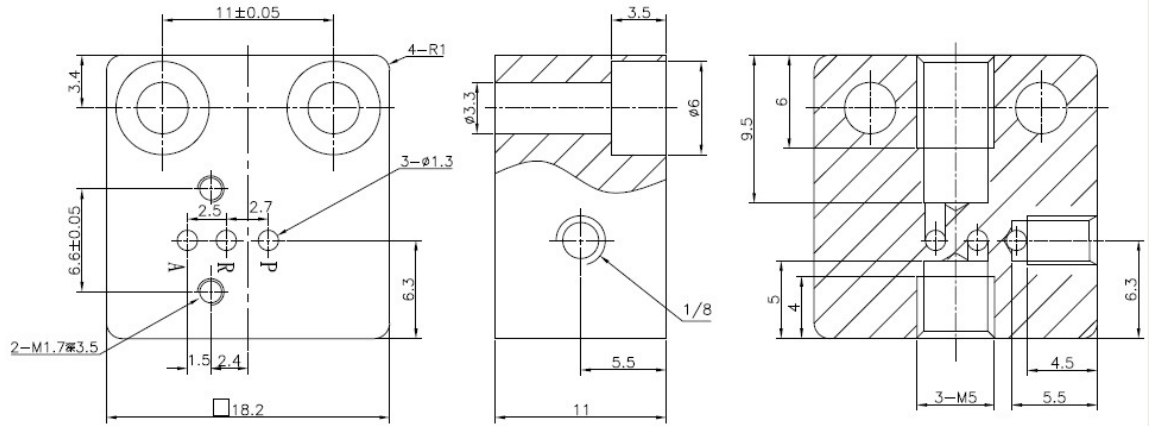
單座尺寸
