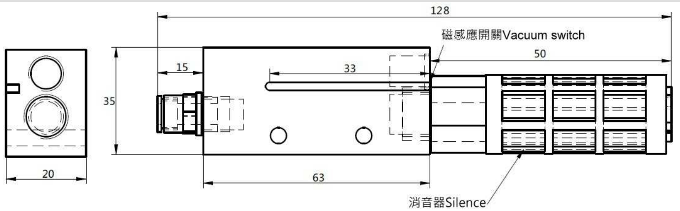
VBR-15
