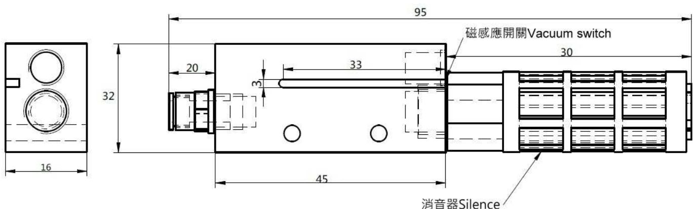
VBR-10
