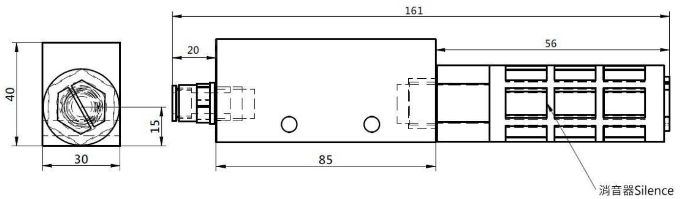
VBR-20
